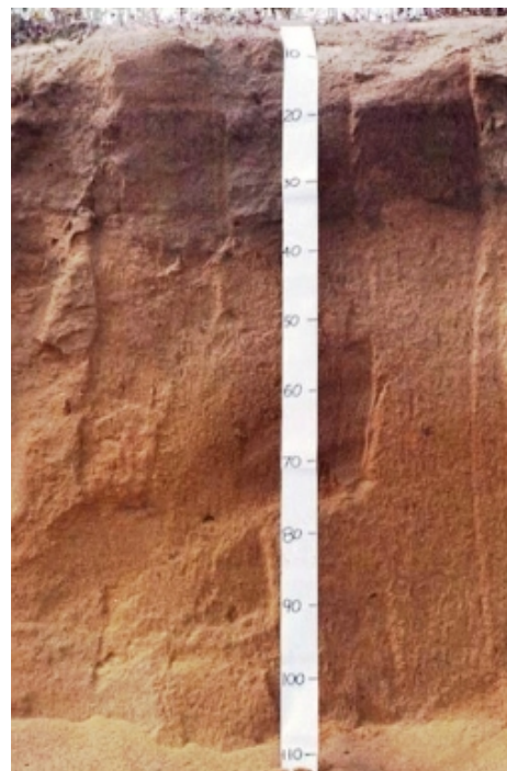
Brown deep sand (Kukerin)
