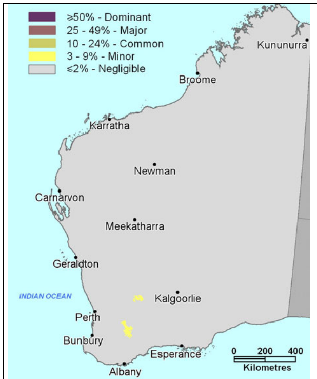
409 Reticulite deep sandy duplex p 74
